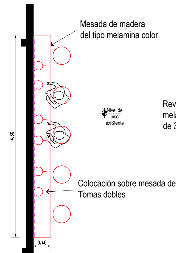
Detalle de mesada
