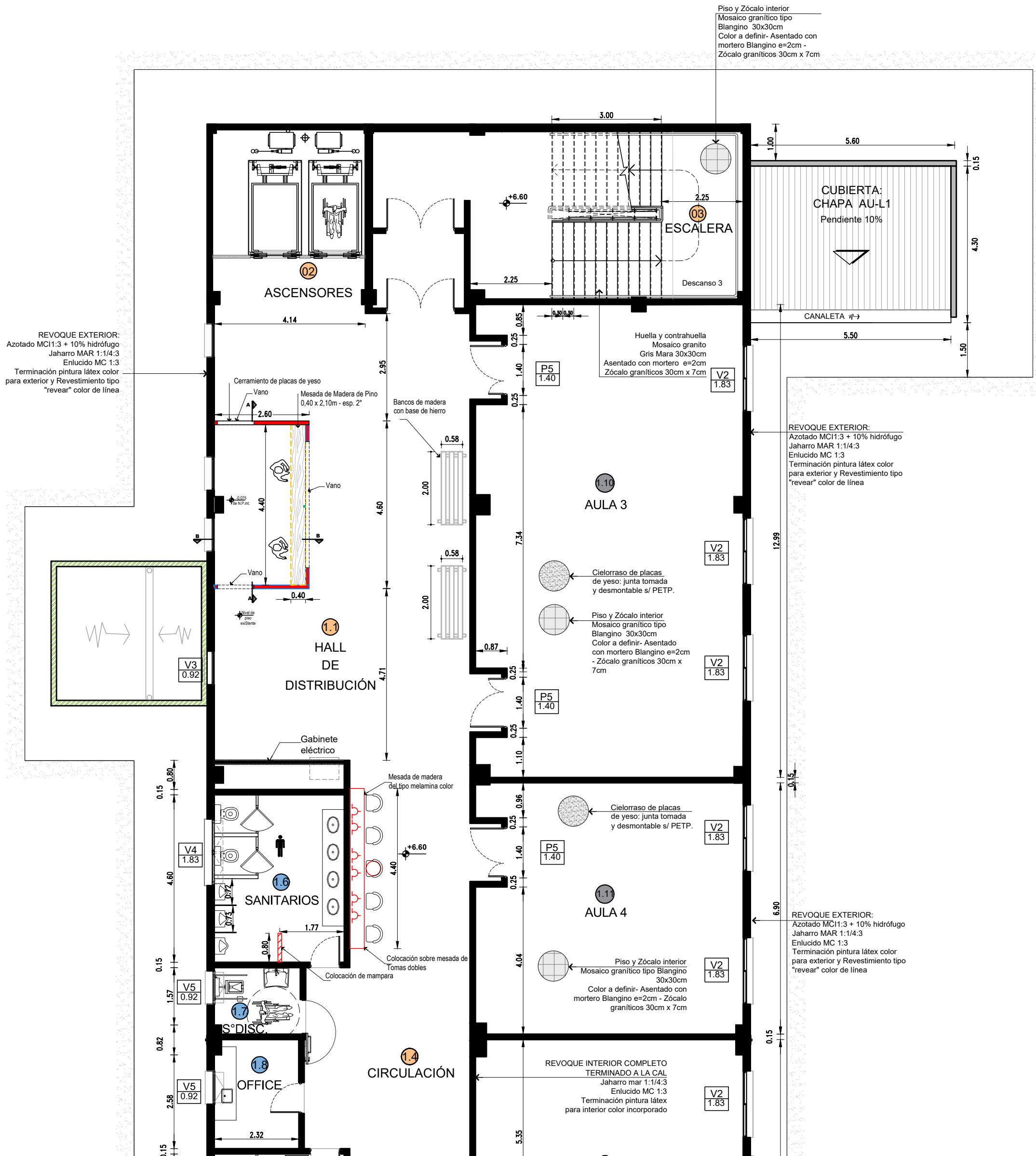
PROPUESTA CENTRO DE ESTUDIANTES_ 1º Piso ESC 1:100
