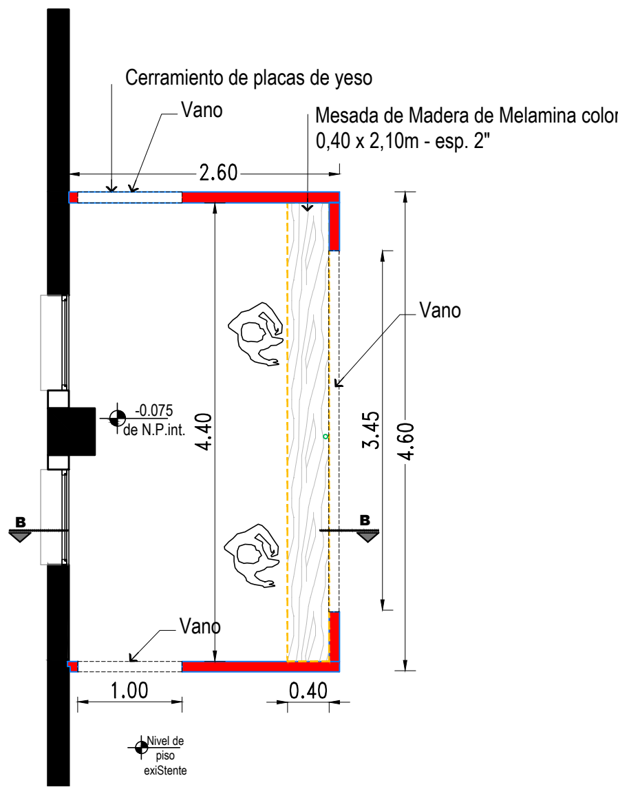
PLANTA CENTRO DE ESTUDIANTE - ESC 1:50
