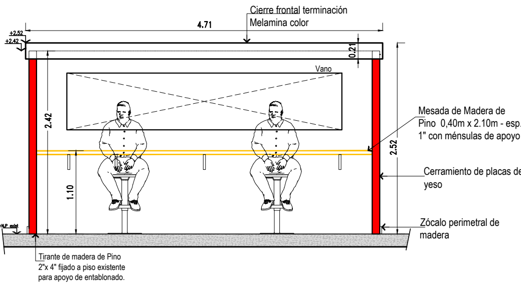
VISTA FRONTAL - ESC 1:50
